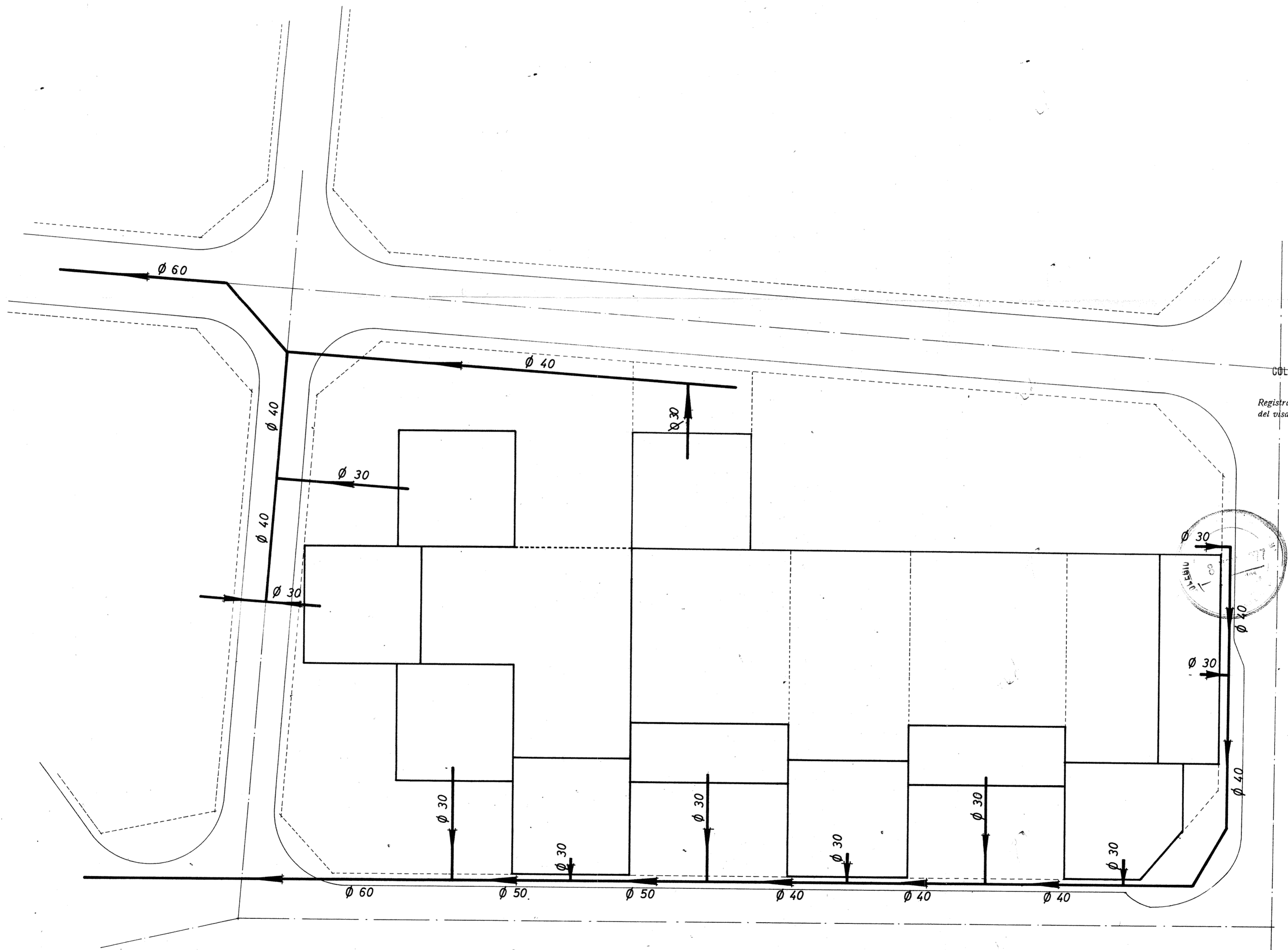
PLANO DE SANEAMIENTO
