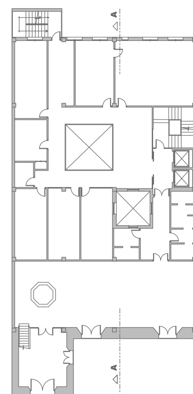
PLANTA SEGUNDA
