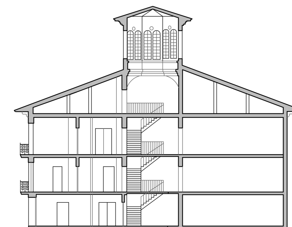
SECCIÓN A-A
