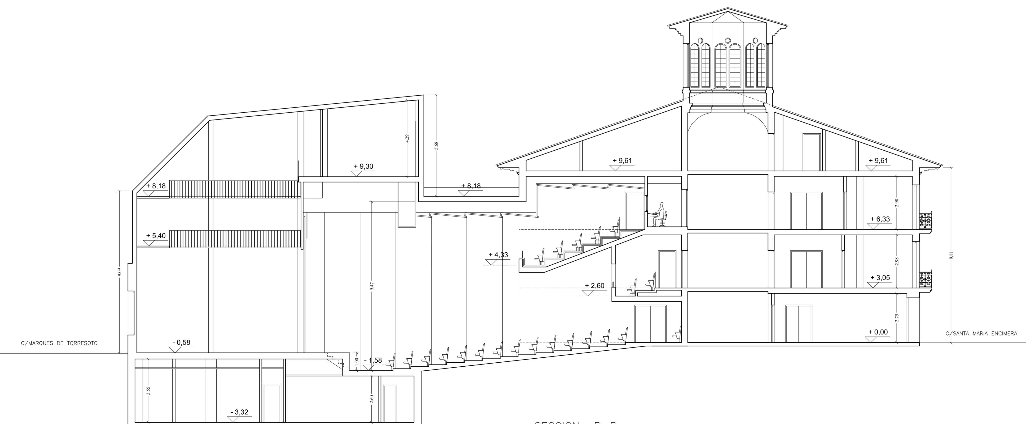
SECCION B-B
