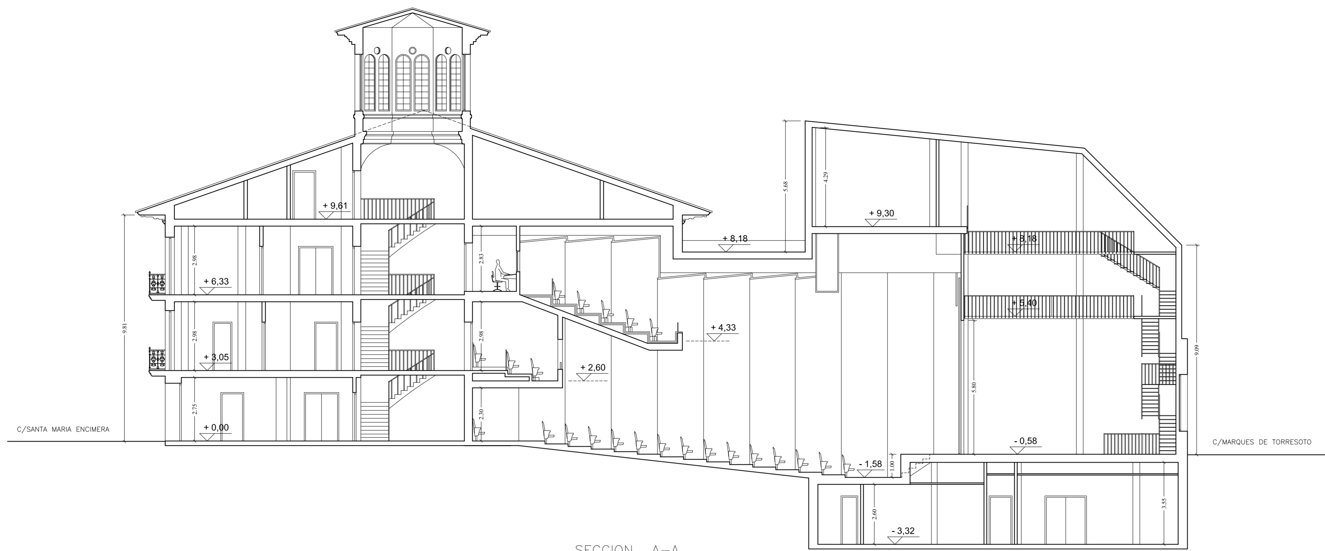
SECCION A-A
